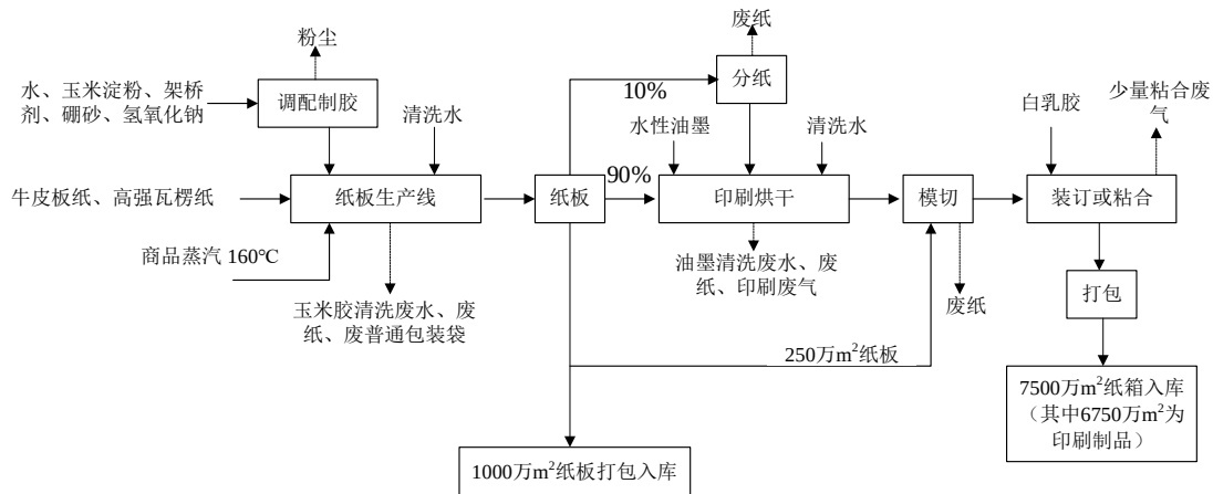
图 3.5-1 本项目纸箱、纸板生产工艺流程及产污环节图
