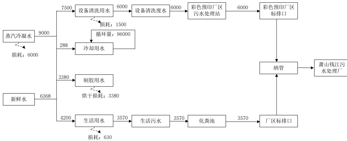
图 3.4-1 本项目水平衡图 单位：t/a
